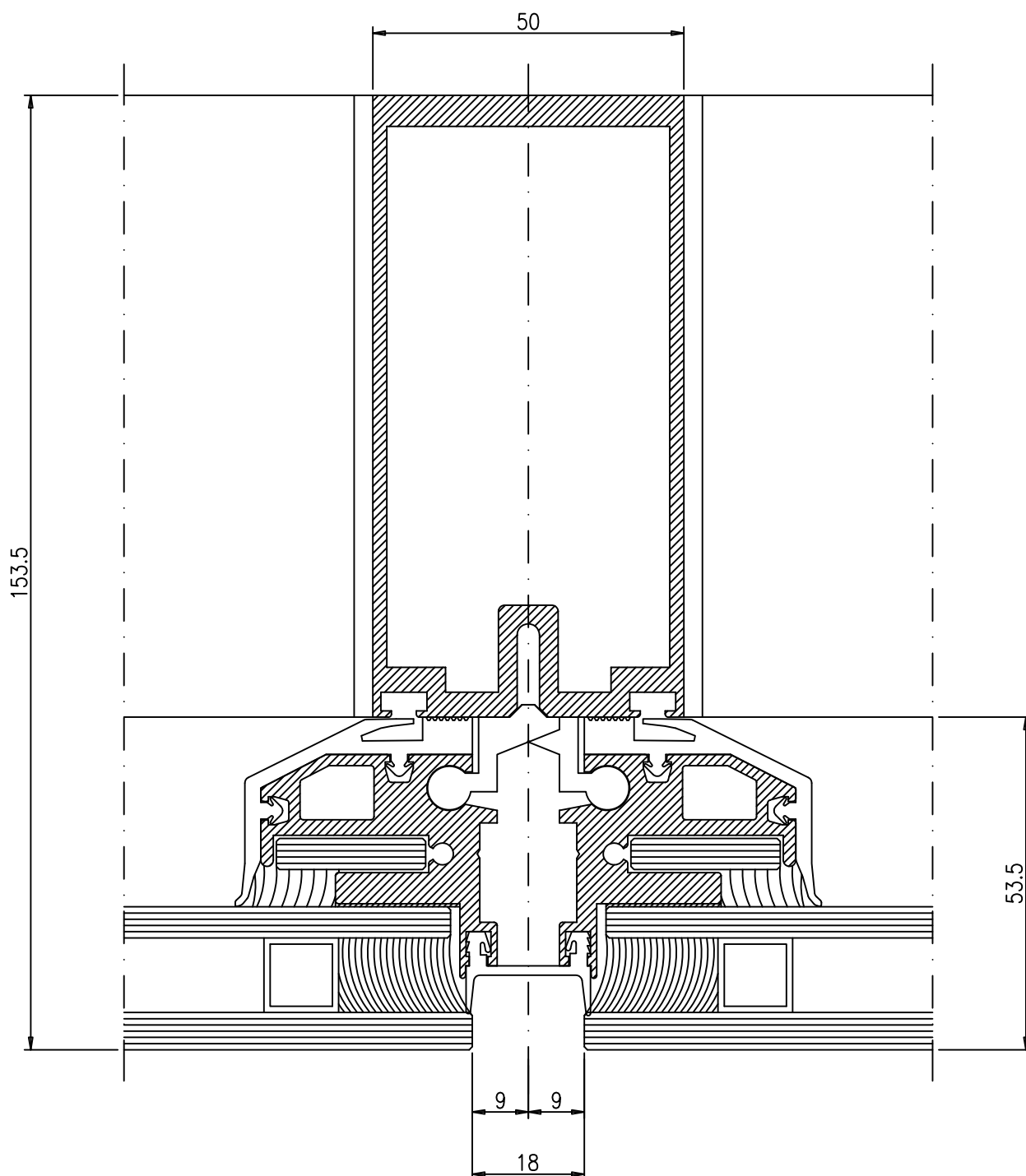
SEZIONE ORIZZONTALE MONTANTE 6771 + ANTA 9006
