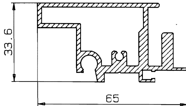
9009 gr/mt 1345 ox mm 265
