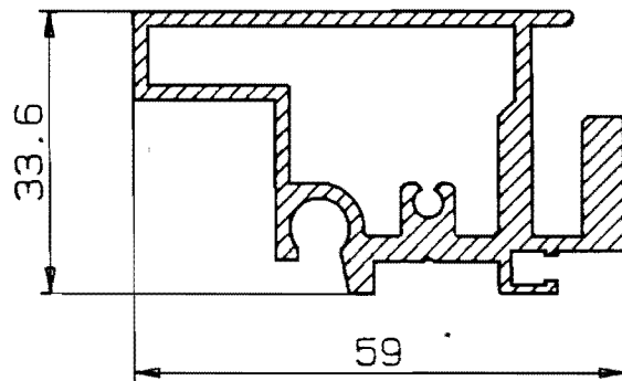
9008 gr/mt 1328 ox mm 256
