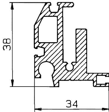
9006 gr/mt 1210 ox mm 235
